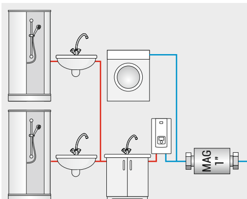
Magnetyzer MAG 1"
